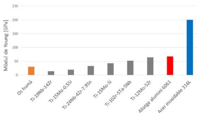
Figura 4: Valors del mòdul de Young de varis aliatges de Titani, comparats amb el valor característic dels teixits ossis humans, un exemple d'aliatge d'Alumini comú i un exemple d'acer inoxidable comú. Modificar els elements d'aliatge permet una modulació eficaç del mòdul de Young dels aliatges de Titani. El mòdul d'elasticitat, o mòdul de Young, és una mesura de la rigidesa d'un material elàstic. De manera molt simplista, el seu càlcul s'efectua mitjançant la mesura de l'allargament uniaxial (en una sola dimensió de l'espai) d'un material quan està sotmès a una certa tensió en la dimensió en qüestió. La complexitat i la informació que pot ser obtinguda mitjançant aquest tipus de mesures essent fora de l'abast d'aquest article, destacarem que la capacitat de modular el mòdul d'elasticitat d'un material permetrà l'obtenció de comportaments variables del mateix quan està sotmès a càrregues mecàniques uniaxials.
