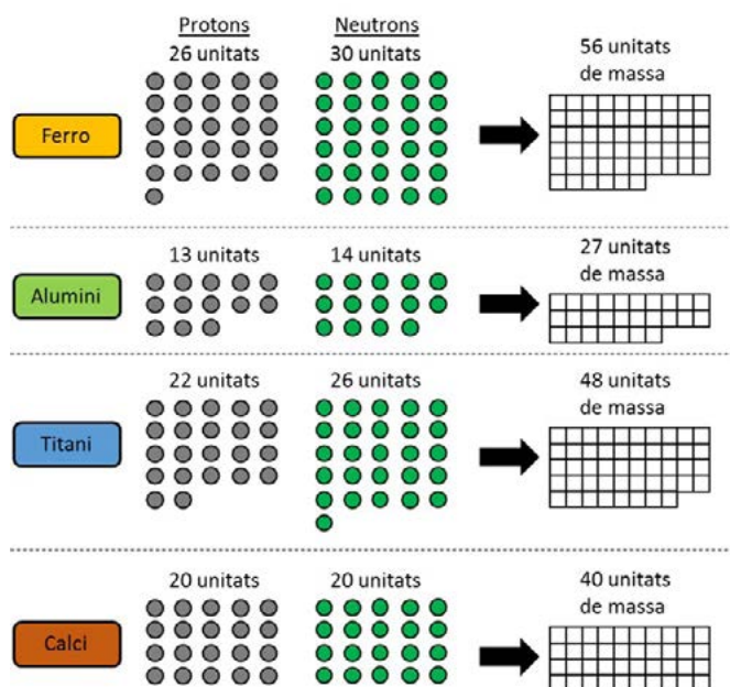
Figura 3: Descripció esquemàtica dels nuclis atòmics dels elements químics següents: Ferro, Alumini i Titani. L'anàlisi pren en compte la forma més estable i naturalment abundant en el planeta Terra d'aquests elements. En primer lloc, 26 protons i 30 neutrons componen el nucli d'un àtom de Ferro, fet que el converteix en un àtom amb 56 unitats de massa. En segon lloc, 13 protons i 14 neutrons componen el nucli d'un àtom d'Alumini, fet que el converteix en un àtom amb 27 unitats de massa. En tercer lloc, 22 protons i 26 neutrons componen el nucli d'un àtom de Titani, fet que el converteix en un àtom amb 48 unitats de massa. Finalment, 20 protons i 20 neutrons componen el nucli d'un àtom de Calci, fet que el converteix en un àtom amb 40 unitats de massa.
