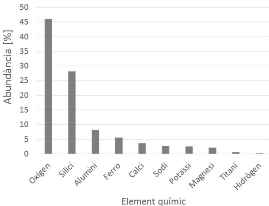
Figura 2: Abundància (en percentatge de pes) de diferents elements químics a l'escorça terrestre. Remarcablement, el Titani representa el novè element més abundant en l'escorça terrestre!
